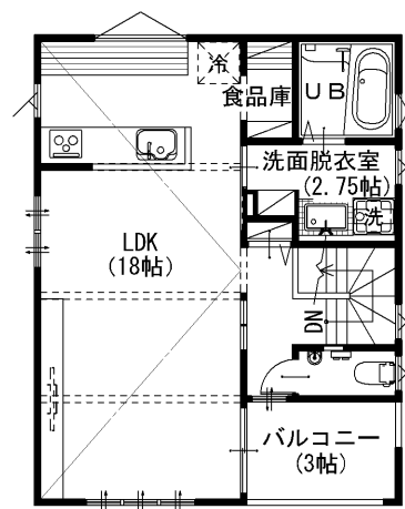
2階 平面図 S:1/100
